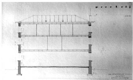
Переріз поверхів
